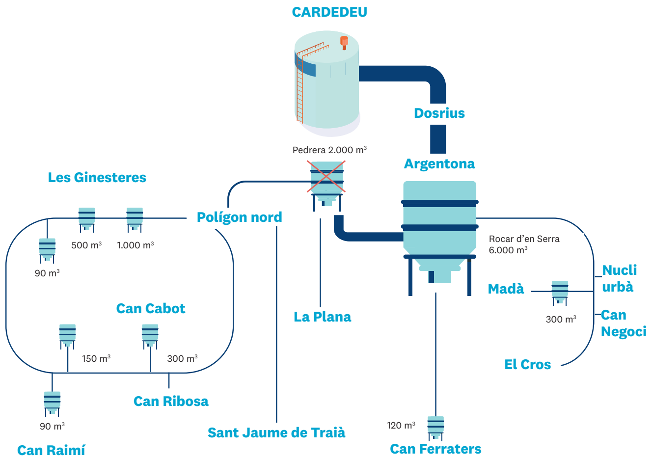
Esquema de la distribució de l'aigua a Argentona. Elaboració pròpia amb dades de la companyia Aigües Argentona.
