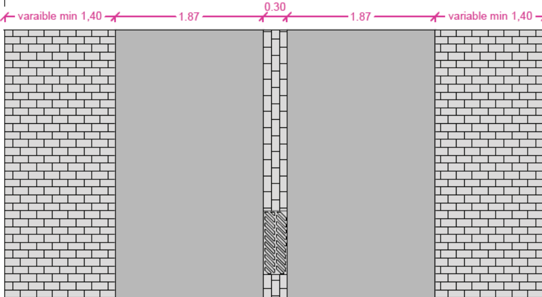
PLANTA TIPUS e: 1/50
