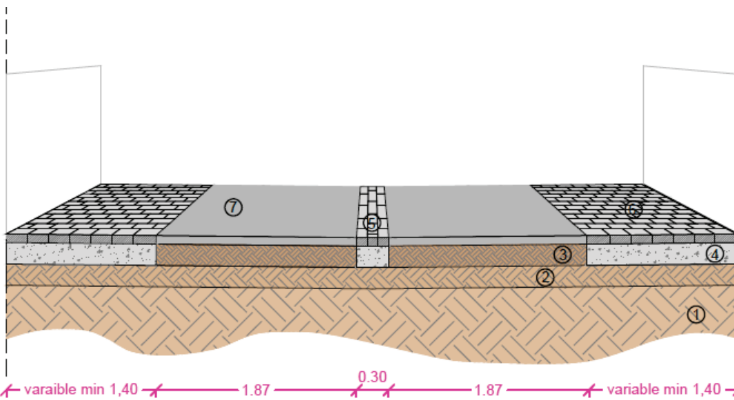
SECCIÓ TIPUS e: 1/50
